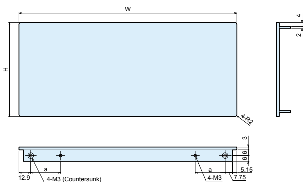
HY Front-Rückplatte und HYR • HYRH Rückplatte HY front / rear panels & HYR • HYRH rear panel
