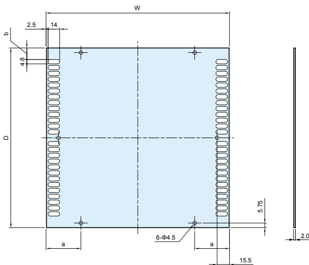
Einzelteilzeichnung - Component Parts Drawings HY • HYR • HYRH Deck-Bodenblech - top / bottom cover
