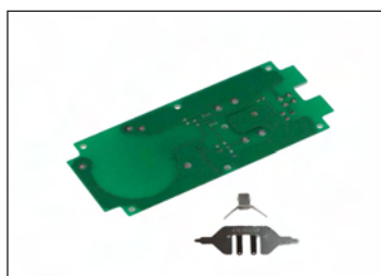
Montierte Kontakte mounted contacts
