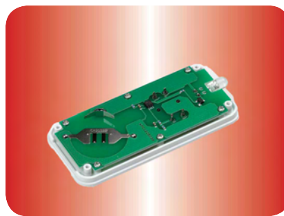
Einbau der Platine auf der oberen Abdeckung
